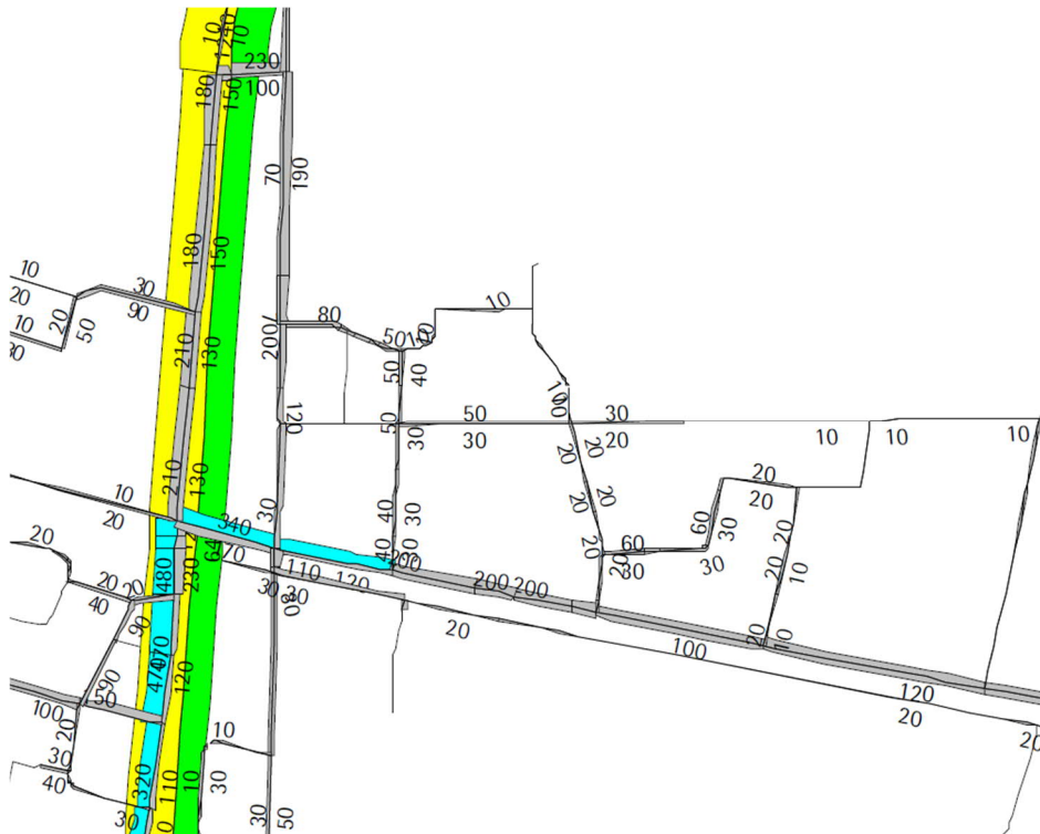
Figuur 20 Verkeersmodel ochtendspits 2020 motorvoertuigen per uur
