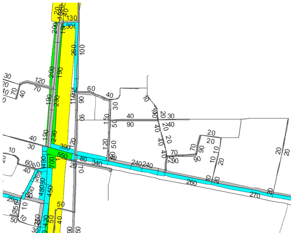
Figuur 21 Verkeersmodel avondspits 2020 motorvoertuigen per uur
